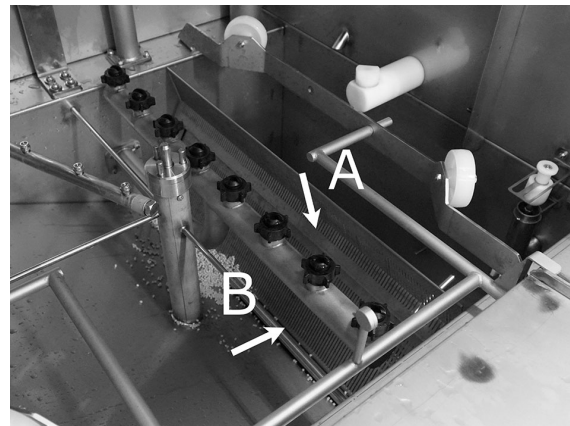
Fig. 37 Granule damper
