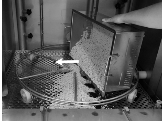
Fig. 5 Granule filling
