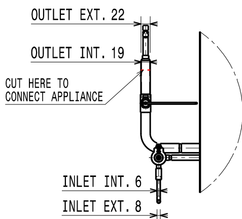
Detail A Scale: 1:9
